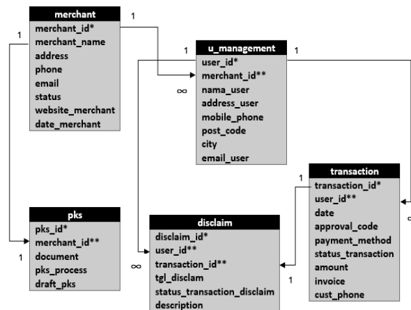
Gambar 4. Relasi Antar Tabel
