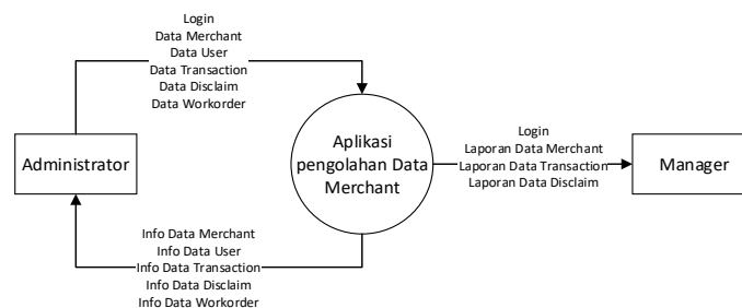
Gambar 5. Diagram Konteks
