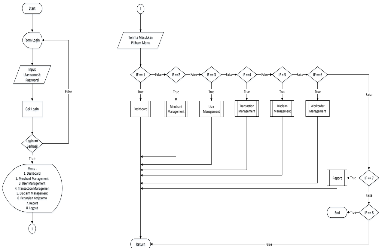
Gambar 2. Flowchart Aplikasi
